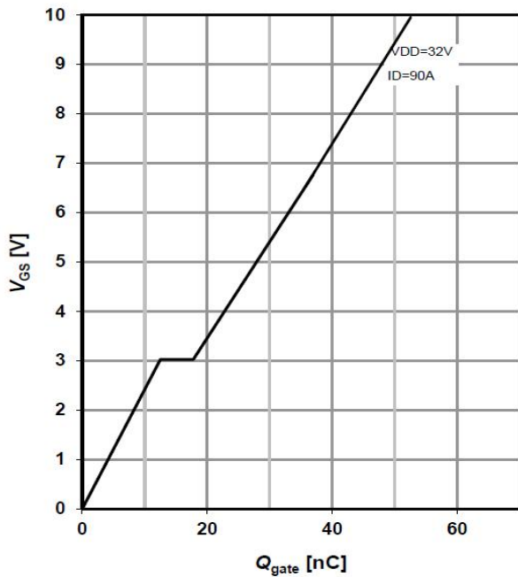
Typ.gate charge
