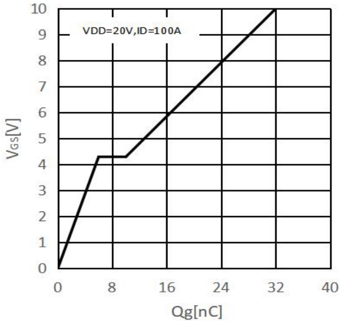
Typ.gate charge
