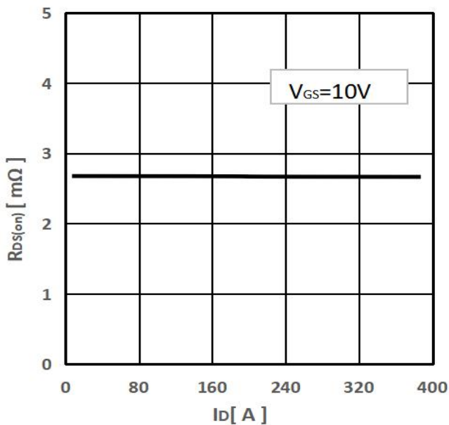
RDS(on) -- ID
